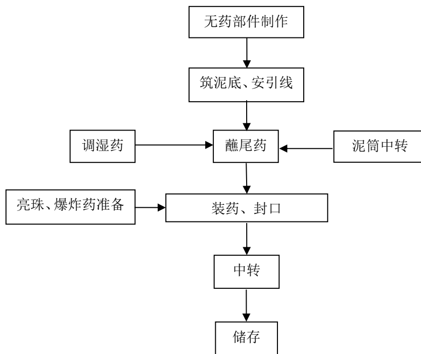
图 2.4-1 效果件内筒（手工装内筒）生产工艺流程图
