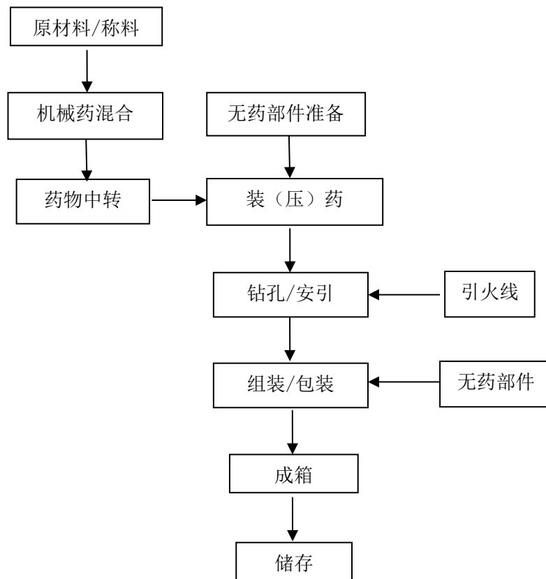
图 2.4-10 架子烟花类产品生产工艺流程图
