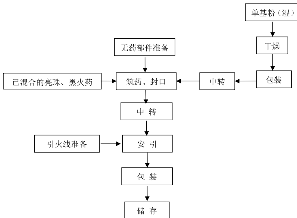
图 2.4-3 吐珠类产品生产工艺流程图
