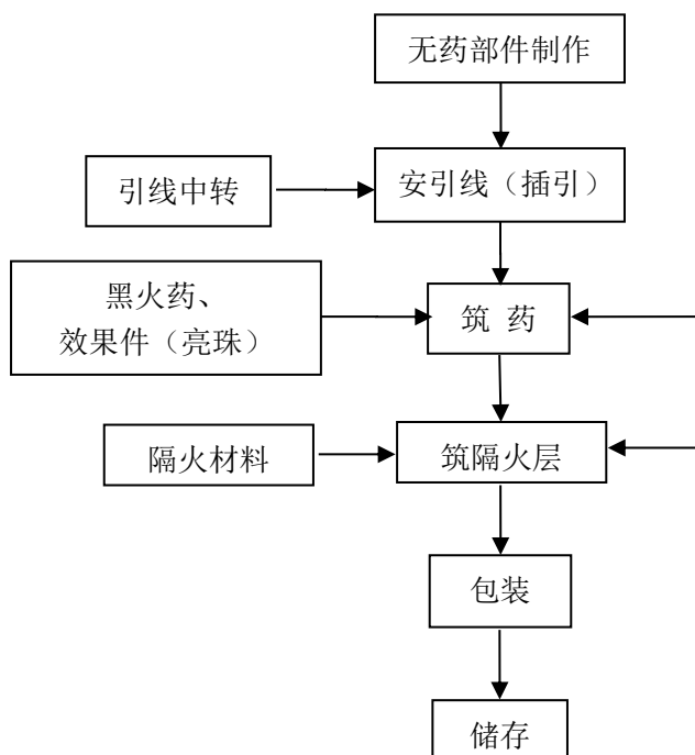
图 2.4-3 吐珠类产品生产工艺流程图
