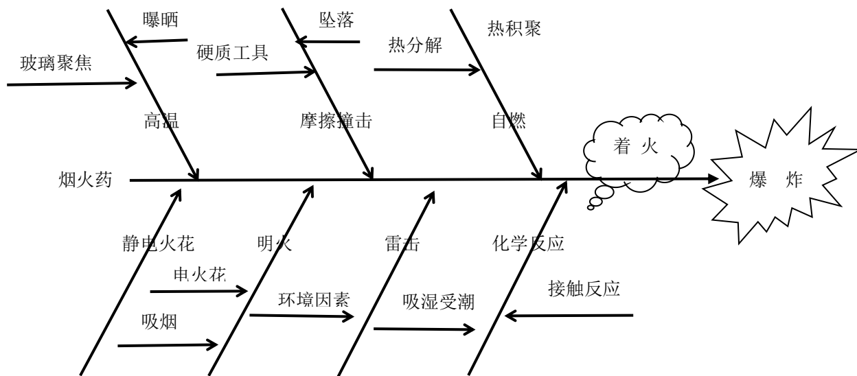
图 3.11-2 烟火药燃烧、爆炸触发条件分析图
