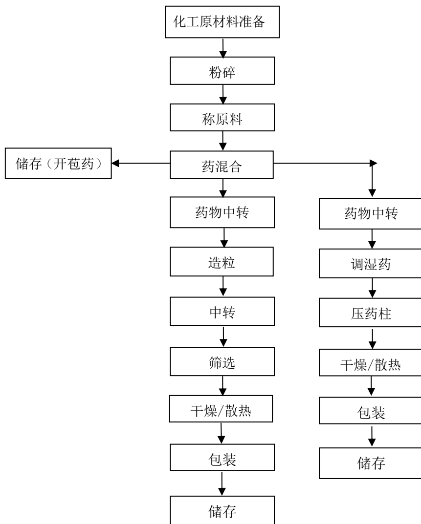
图 2.4-2 药物裸药效果件（亮珠、药柱、开苞药）生产工艺流程图
