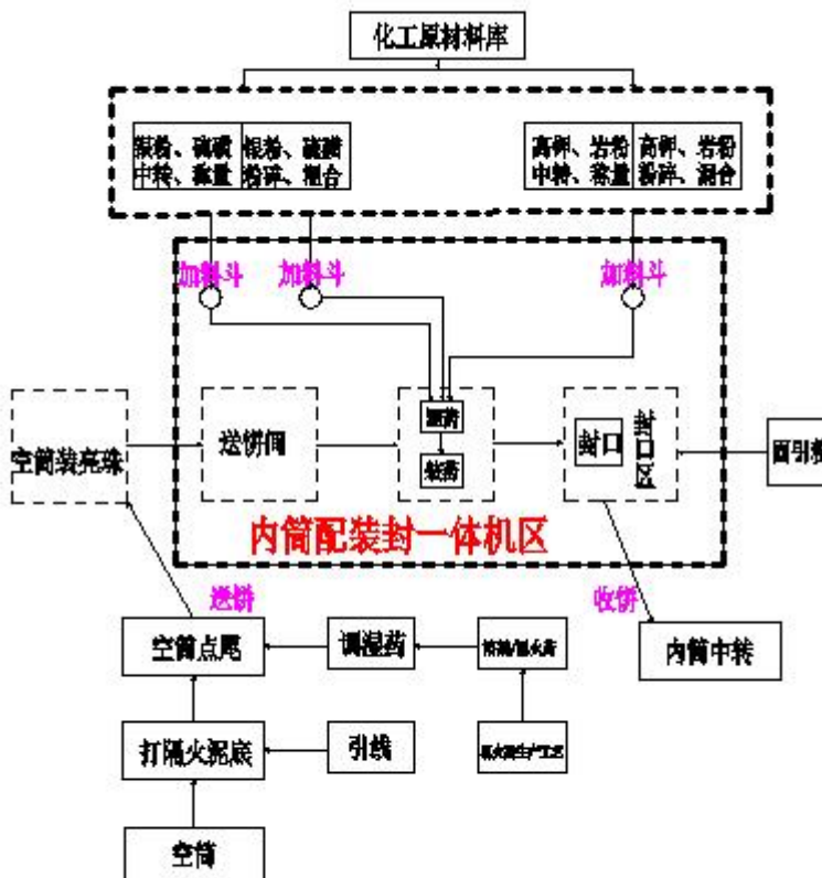
组合烟花内筒装药一体机内筒生产工艺流程图
